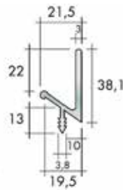
Profil poignée type 901189
