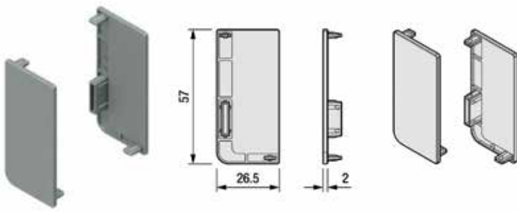
Embout Gola L Led - par kit (2 pièces)
