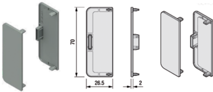
Embouts Gola C Led - par set (2 pièces)
