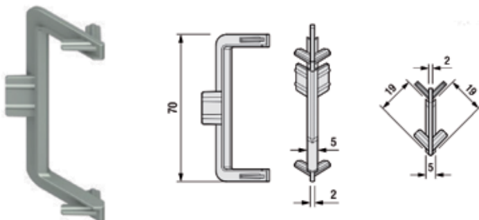
Pièce d'angle extérieure Gola C Led
