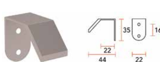
Bouton en zamac type 3600
