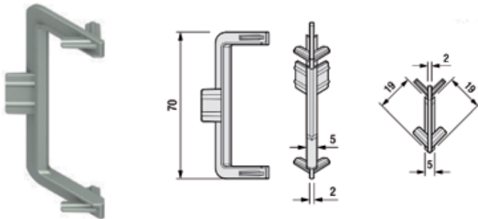
Pièce d'angle extérieure Gola C
